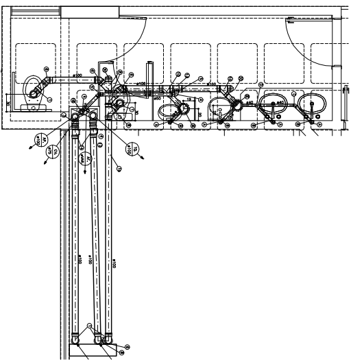
E WC COLETIVO MASCULINO 20 ESCALA 1:20 (1° PRANDIO)
