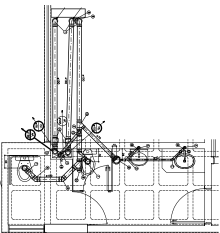
E WC COLETIVO FEMININO 19 ESCALA: 1:20 (1ª PAVIMENTO)
