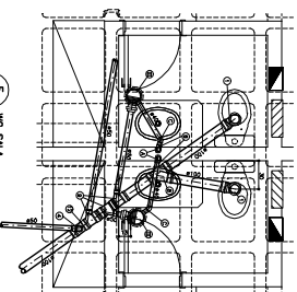
E WIC SALA 22 ESCALA: 1:20 (1° PLANTENO)
