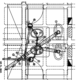
E MC SALA 21 ESCALA, 1:100 (1° PRINCIPAL)
