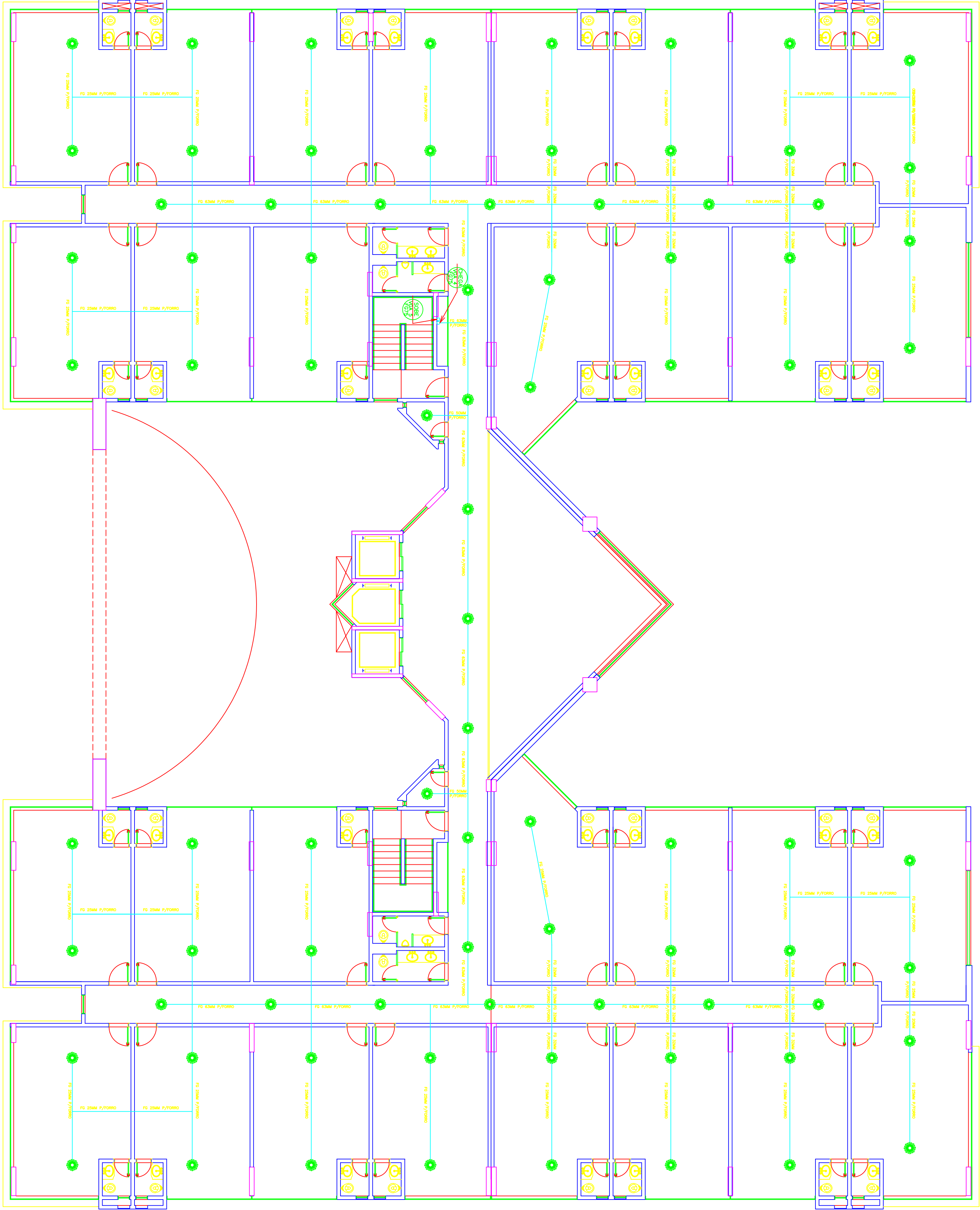
PLANTA BAIXA DO 2º PAVIMENTO
