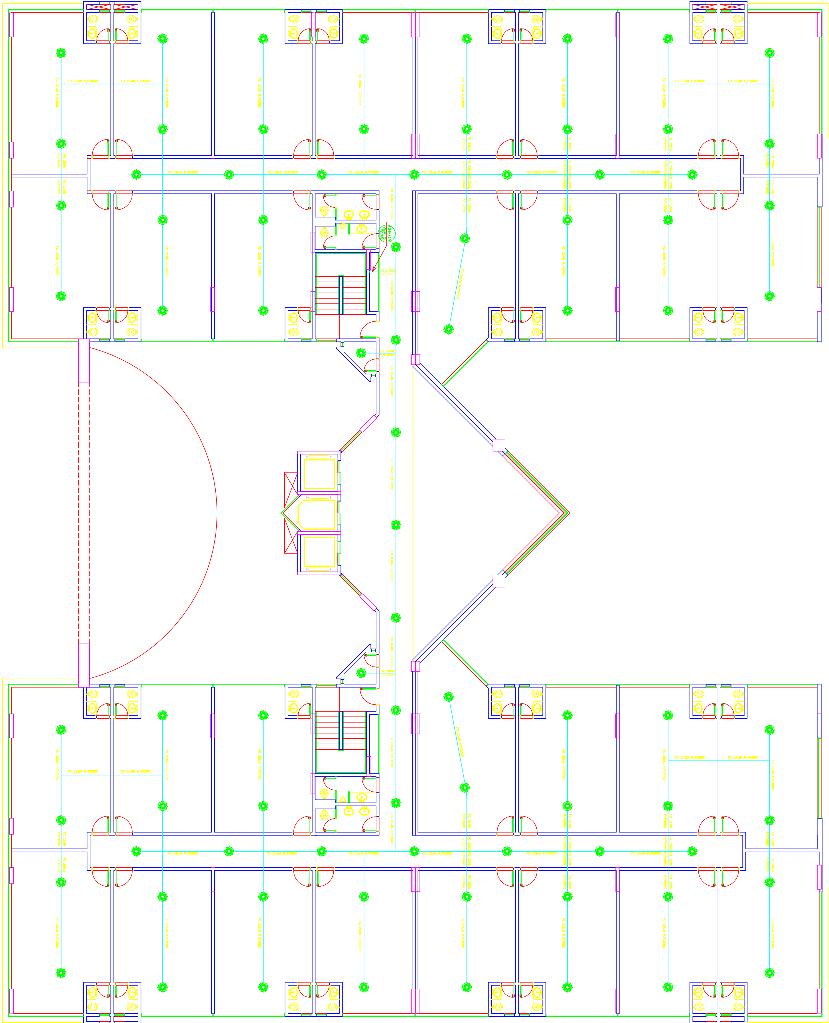
PLANTA BAIXA DO 3º PAVIMENTO
