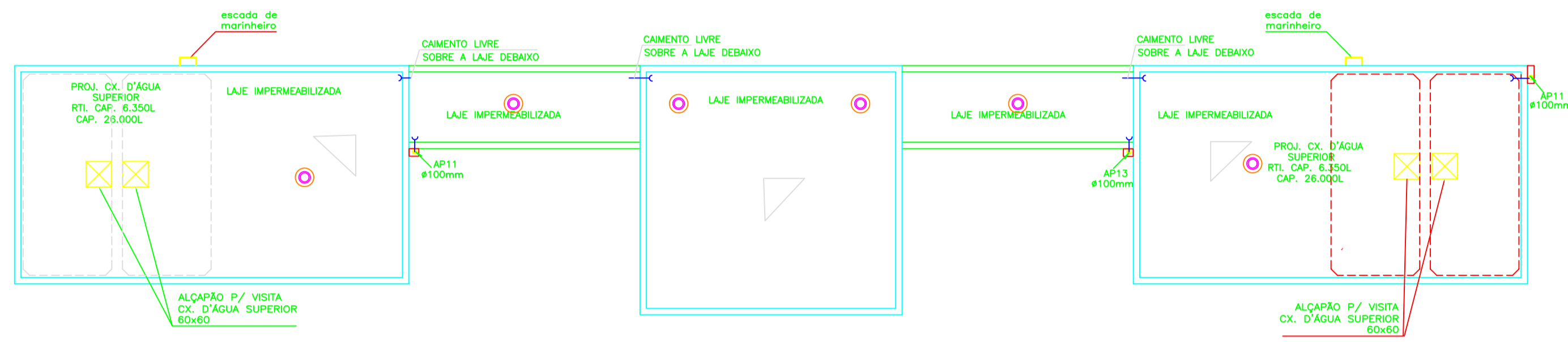
COBERTURA DA CX. D'ÁGUA E CASA DE MÁQ. ESCALA 1:100
