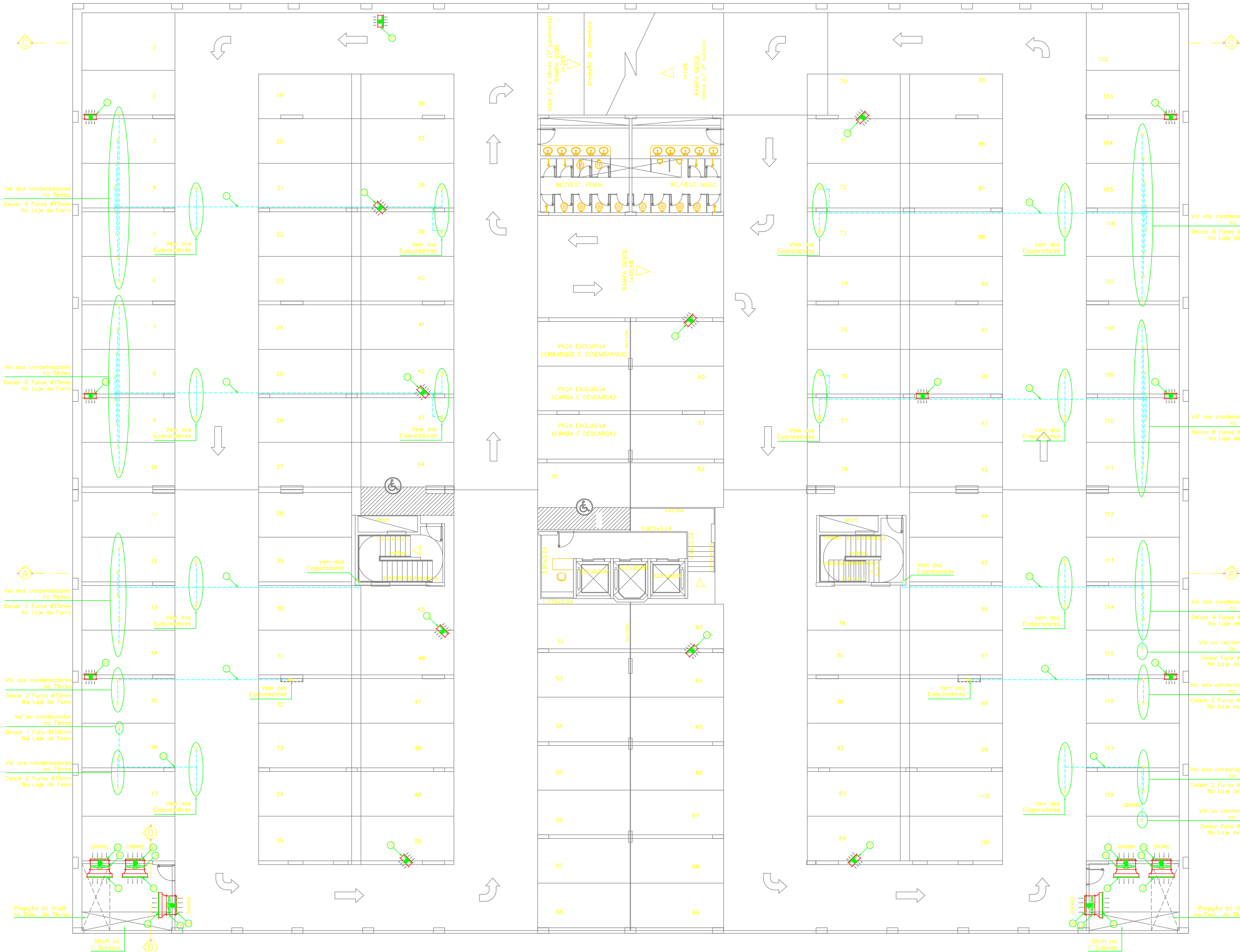
PLANTA BAIXA 1º SUBSOLO ESCALA 1:100
