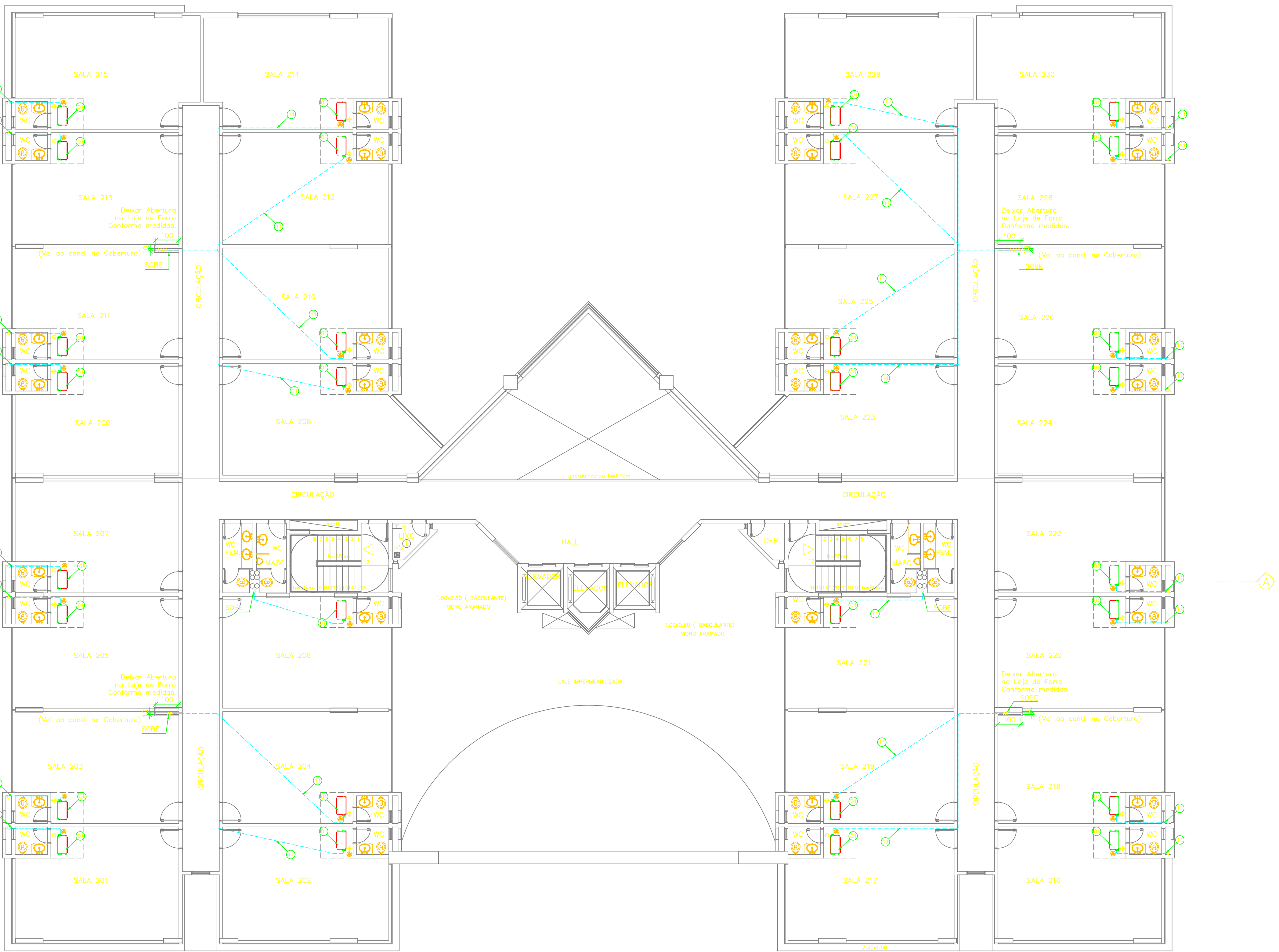
PLANTA BAIXA DO 2º PAVIMENTO ESC 1:100
