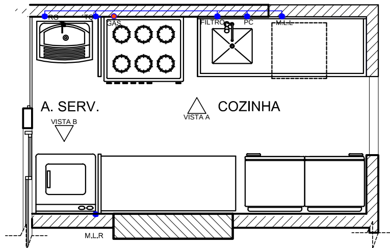
COZINHA PLANTA BAIXA
