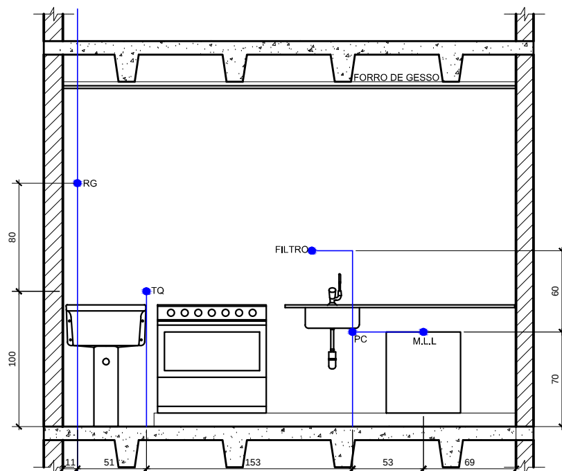
COZINHA VISTA A
