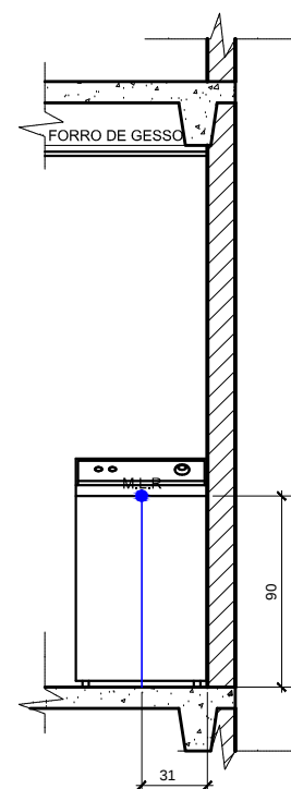
Ê. SERVIÇO VISTA B - ponto M.L.R.
