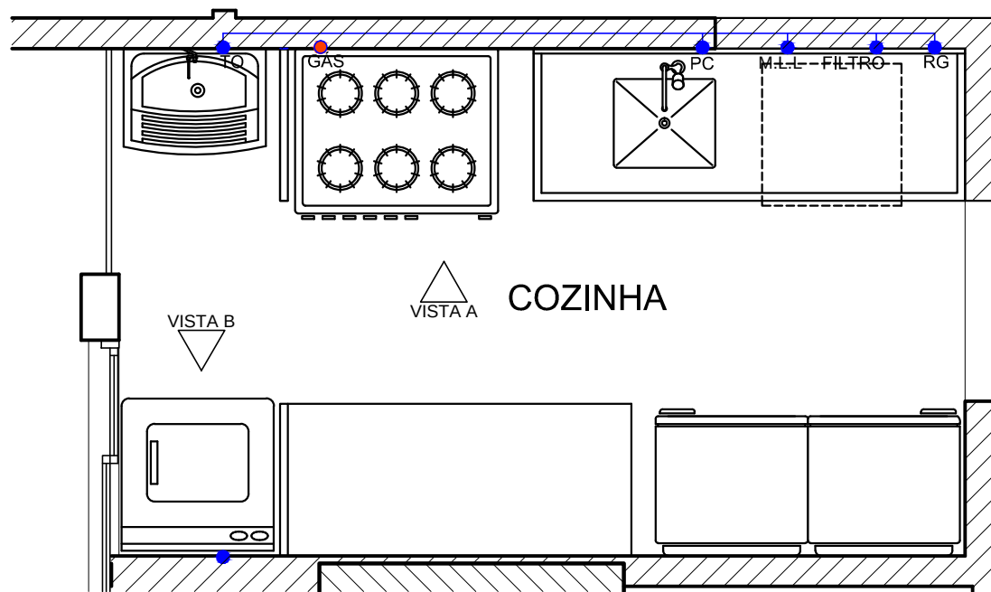
COZINHA PLANTA BAIXA
