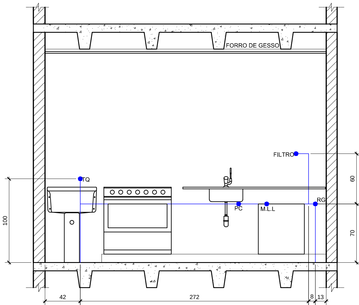
COZINHA VISTA A
