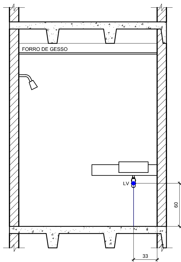
BANHO SUÍTE VISTA B
