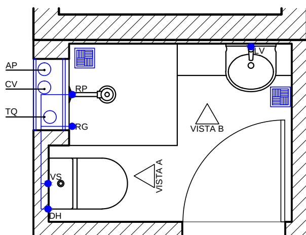
BANHO SUÍTE PLANTA BAIXA
