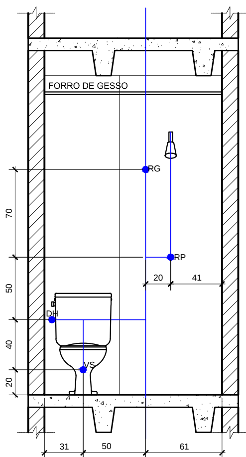
BANHO SUÍTE VISTA A
