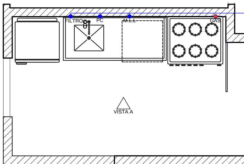
COZINHA PLANTA BAIXA
