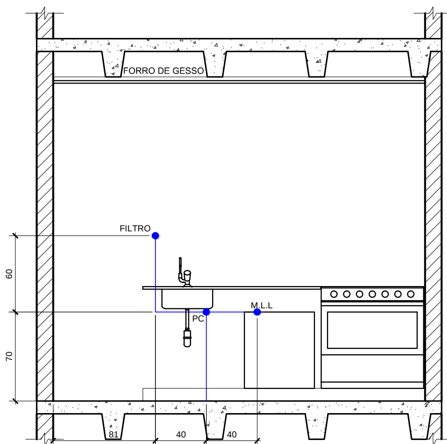
COZINHA VISTA A
