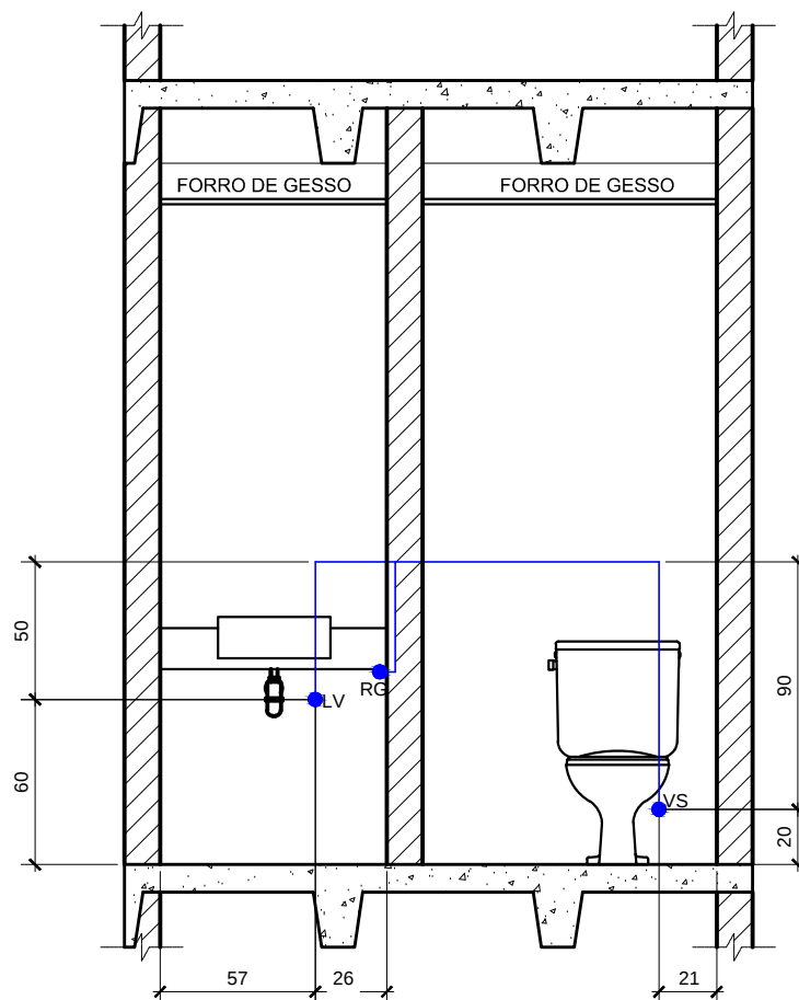
BANHO LAVABO VISTA A
